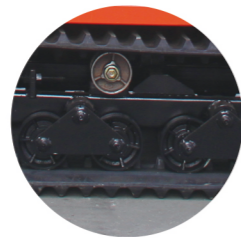
浮动轮系 Floating gear train
